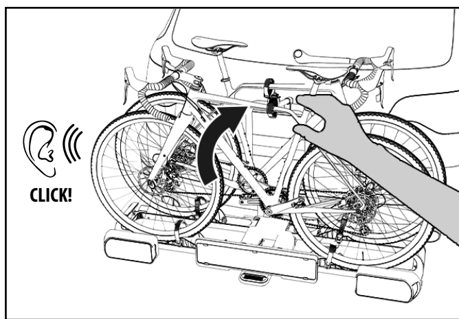
Figura 31: Risollevarlo del portabici
