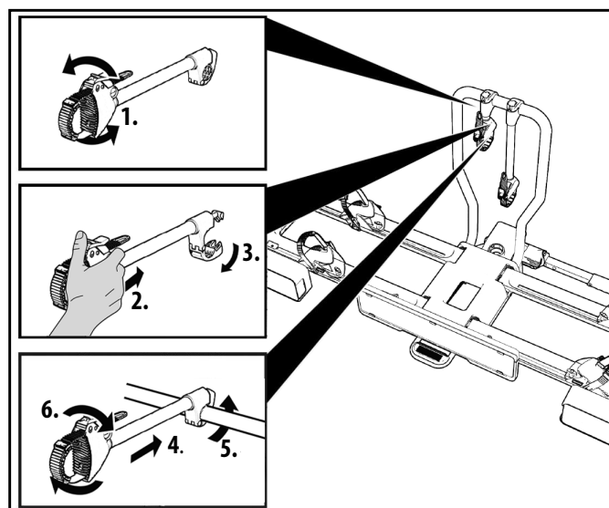
Figura 9: Montaggio bracci di fissaggio
