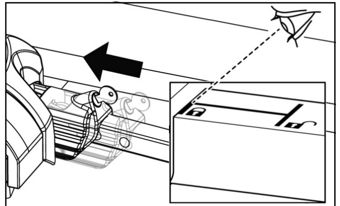
Figure 13: Verrouillage du système de fermeture rapide
