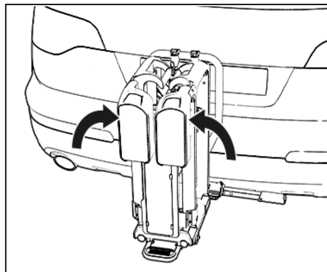
Figura 34: Chiusura del portabicycle
