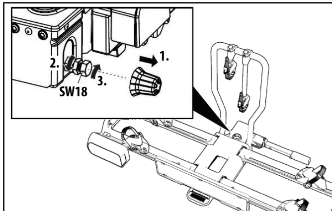
Bild 15: Einstellen des Schnellverschlusses
