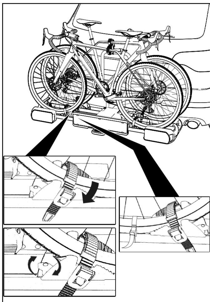
Figura 26: Fissaggio della ruota anteriore, seconda bicicletta
